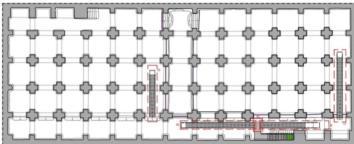
Figura 14 - Pianta a quota +18,00 con indicazione dell'area oggetto di intervento del progetto FSC
