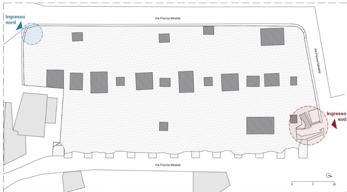
Figura 13 - Pianta delle coperture della Piscina Mirabilis – intervento del progetto PON in corso sugli ingressi sud e nord
