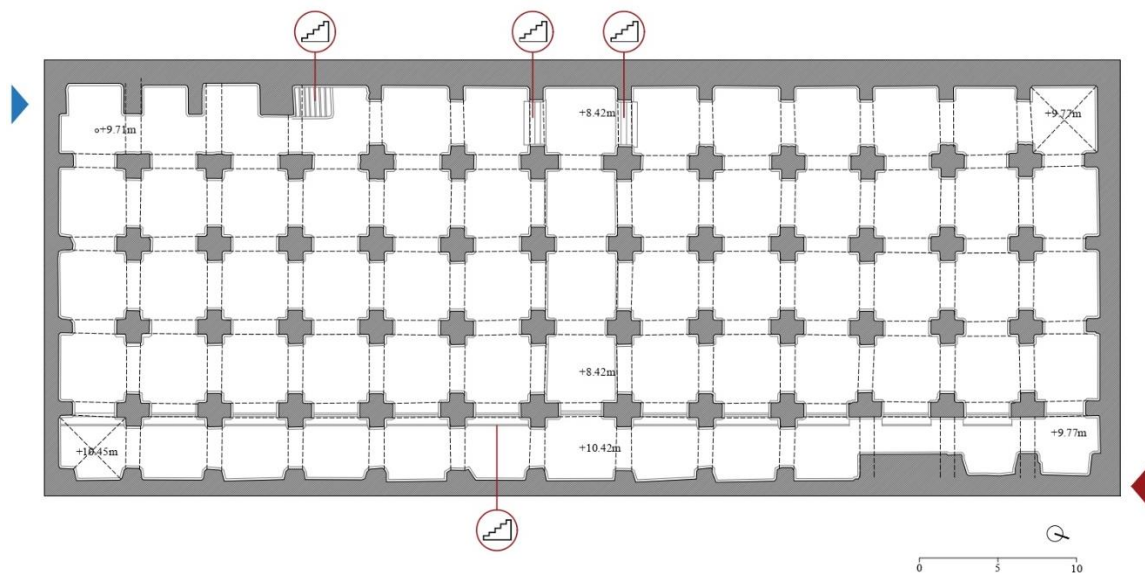
Figura 17 – Pianta a quota +11,00
