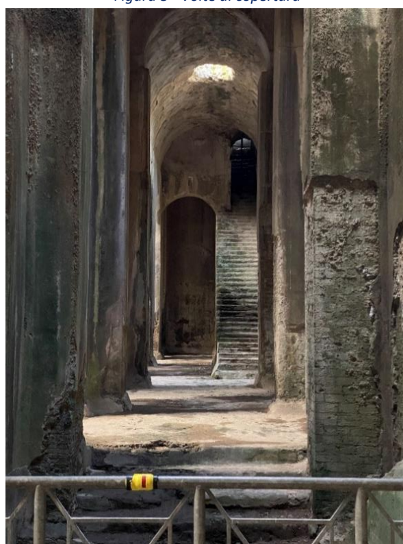
Figura 5 – Ingresso nord (di servizio)
