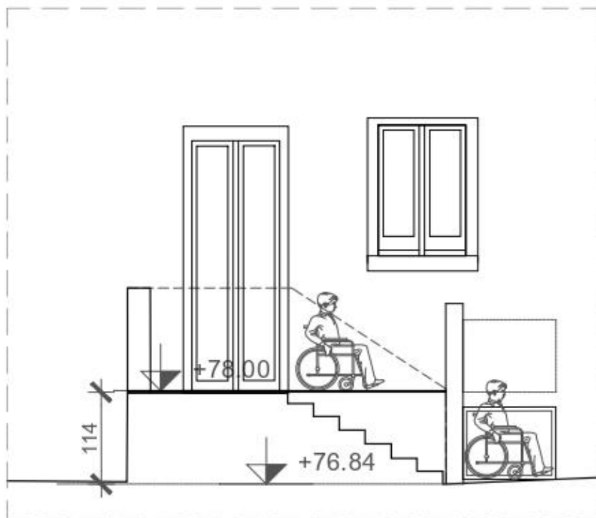
Figura 24 - Schema posizionamento pedana e piattaforma elevatrice
