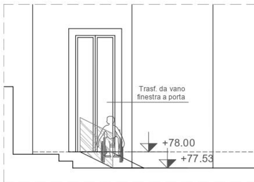
Figura 23 - Schema passerella in prospettiva
