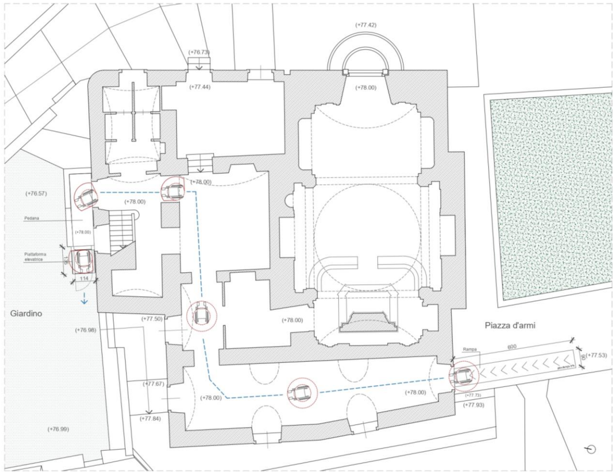
Figura 22 – Schema di posizionamento della passerella e della piattaforma elevatrice
